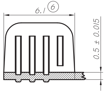
CORTE A-A
